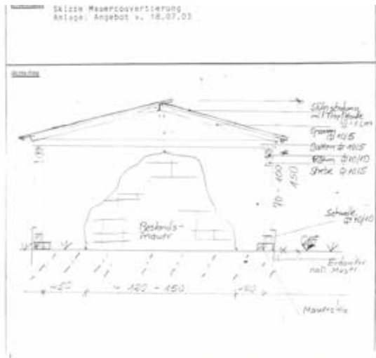
Zeichnung und Musterentwurf Schutzdach für historisches Mauerwerk
